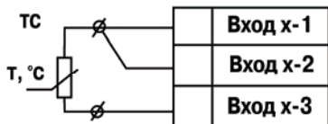
Рис. Б.1. Схема подключения термометра сопротивления
