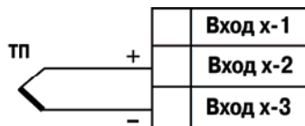
Рис. Б.2. Схема подключения термоэлектрического преобразователя
