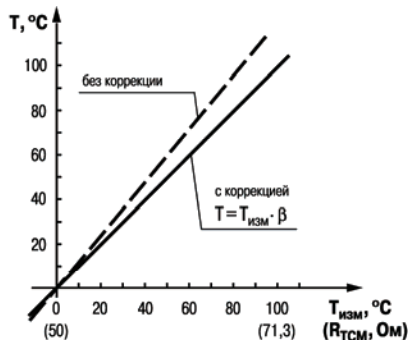
Рис. 3.4. Коррекция «наклон характеристики»
