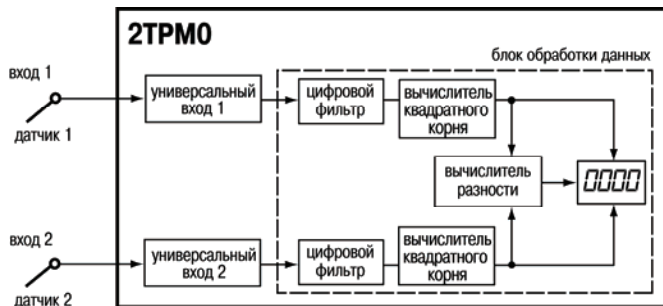
Рис. 3.1. Структурная схема прибора
