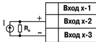
Рис. Б.4. Схема подключения активного датчика с токовым выходом 0 ... 5, 0 ... 20 или 4 ... 20 мА
