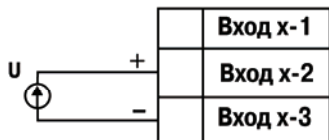
Рис. Б.3. Схема подключения активного датчика с выходом в виде напряжения -50 ... 50 мВ или 0 ... 1 В
