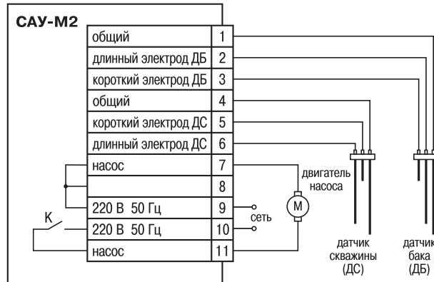
Рис. Б. 1. Подключение САУ-М2 при использовании для заполнения резервуара с помощью погружного насоса с защитой от "сухого хода"
