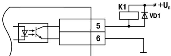
Рисунок 3.6 – Схема подключения нагрузки к ВУ типа К
