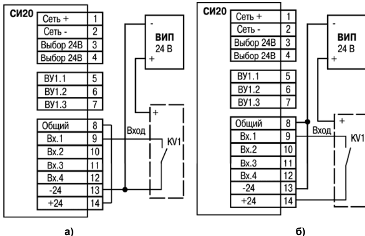
Рисунок 3.2 – Подключение к входу коммутационных устройств: а) при работе с п-р-п датчиками; б) при работе с р-п-р датчиками
