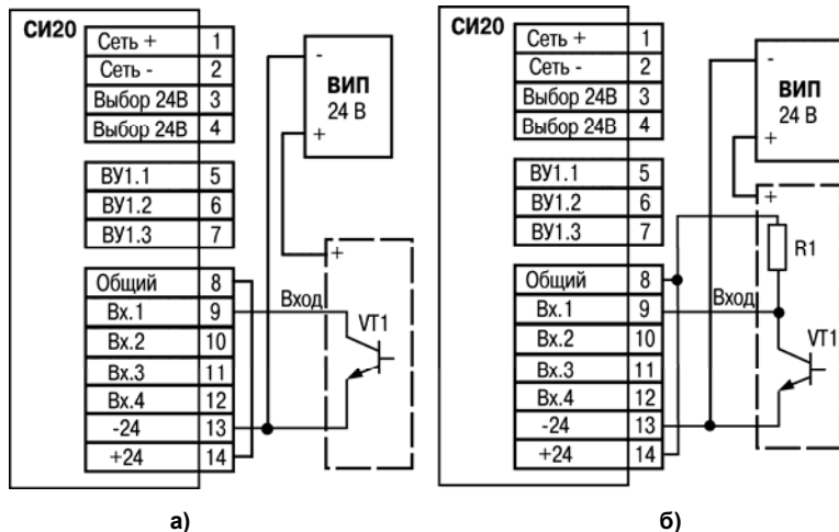
Рисунок 3.3 – Подключение датчиков, имеющих на выходе транзистор p-р-п типа с открытым коллекторным входом:
