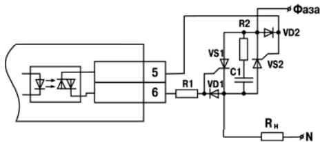
Рисунок 3.8 – Схема подключения к ВУ типа С двух тиристоров, подключенных встречно-параллельно
