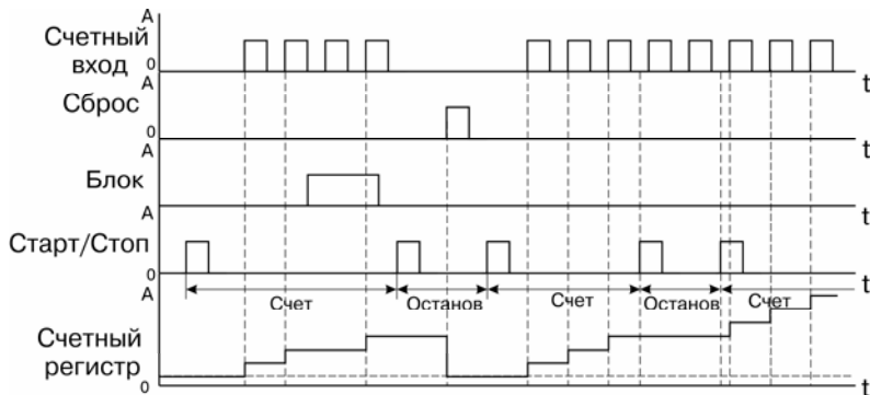
Рисунок 3.11 – Диаграмма работы прибора
