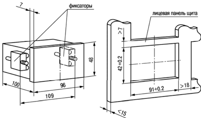
Рисунок А.2 – Прибор щитового крепления Щ2
