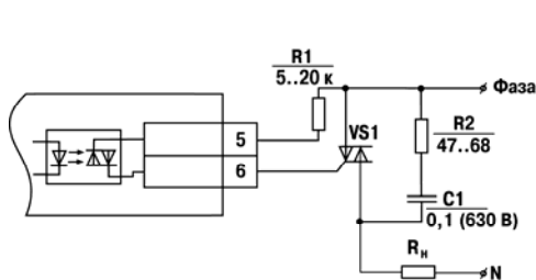
Рисунок 3.7 – Схема подключения силового симистора к ВУ типа С
