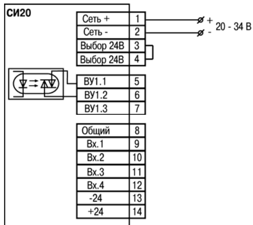
Рисунок Б.2 – Схема подключения прибора СИ20-У.Х.С от сети постоянного напряжения
