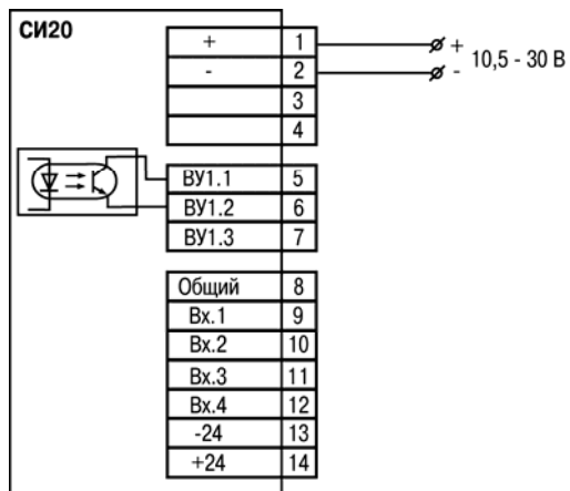
Рисунок Б.3 – Схема подключения прибора СИ20-24.Х.К
