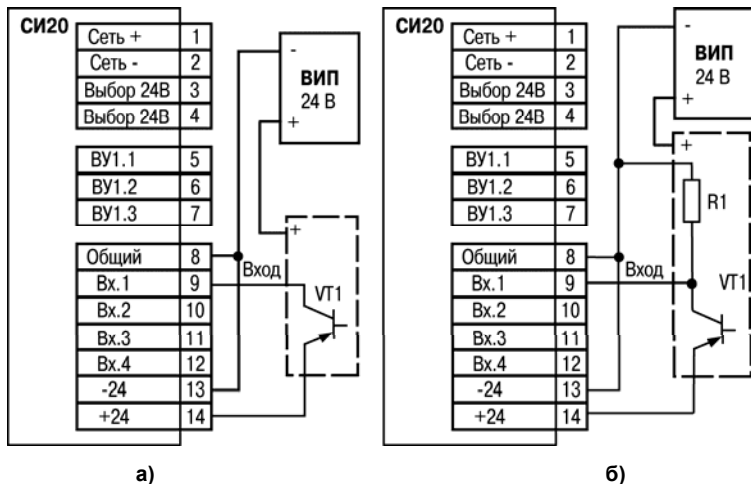
Рисунок 3.4 – Подключение к входу датчиков, имеющих на выходе транзистор р-п-р типа: а) пассивный датчик; б) активный датчик
