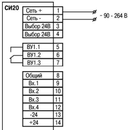
Рисунок Б.1 – Схема подключения прибора СИ20-У.Х.Р от сети переменного тока
