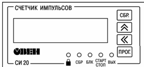
Рисунок 3.10 – Внешний вид лицевой панели прибора для корпуса и щитового (Щ2) крепления
